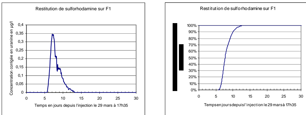
Figure 4 : Courbe de restitution à la Courbe cumulative à la source F1 source F1
