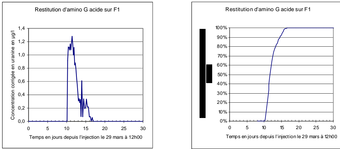
Figure 3 : Courbe de restitution à la source F1 Courbe cumulative à la source F1
