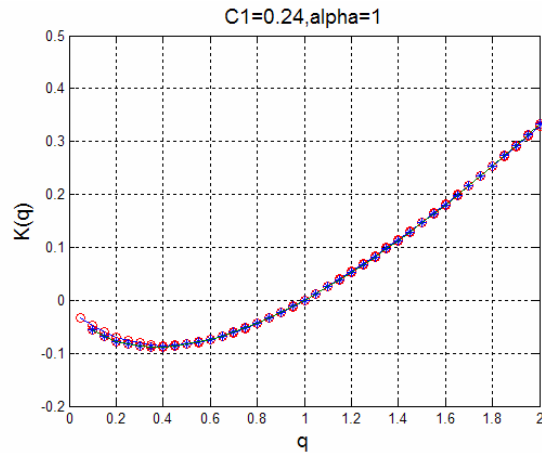
Fig. 4. Spectre multifractale
